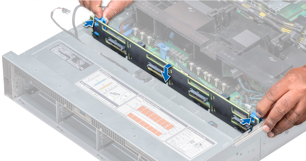
Figure 66. Installation du fond de panier de disque dur
