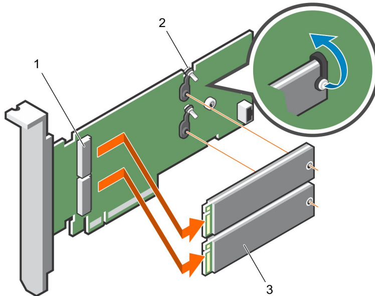
Figure 82. Retrait du module de disque dur SSD M.2
