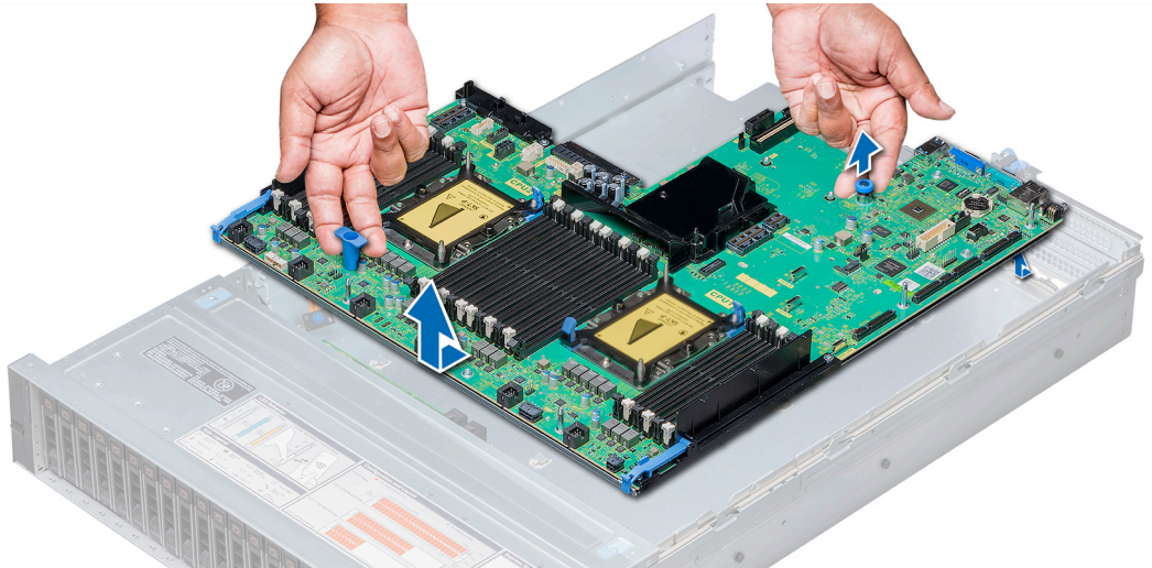
Figure 71. Retrait de la carte système
