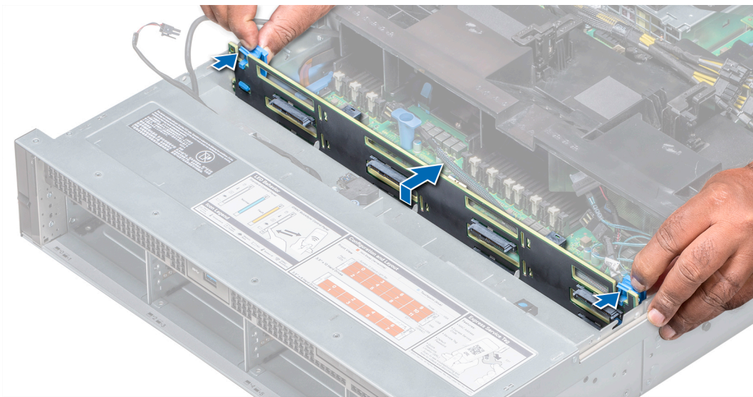
Figure 65. Retrait du fond de panier de disque dur
