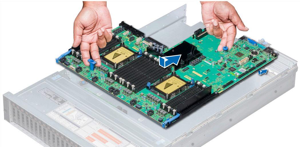
Figure 72. Installation de la carte système
