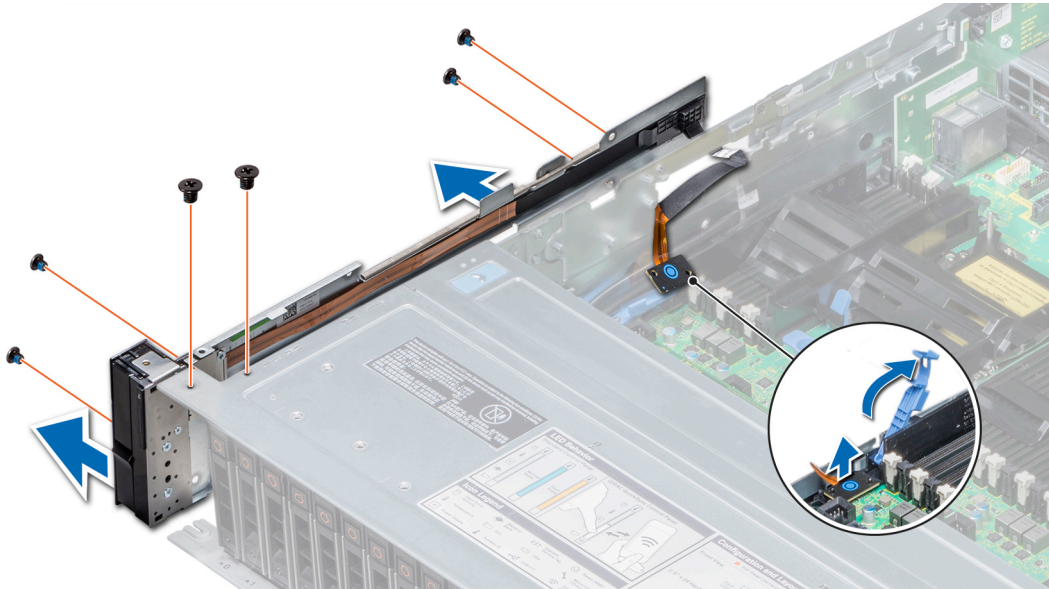
Figure 74. Retrait du panneau de commande gauche
