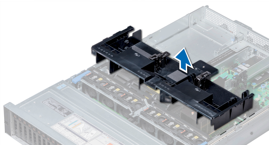
Figure 22. Retrait du carénage d'aération
